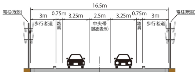
【標準断面図】
