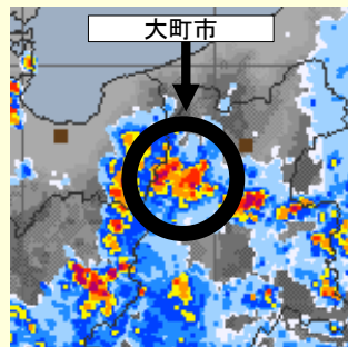
大町市付近の雨雲レーダー画像図 (平成28年8月1日)
