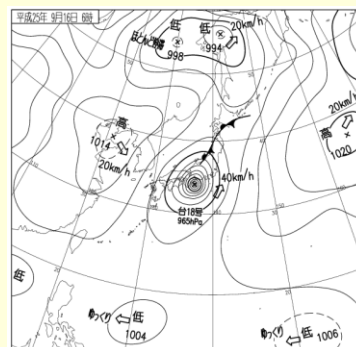
台風の影響で大町市で降水量が多くなった気圧配置 (左：平成23年9月、右：平成25年9月)
