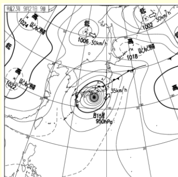
台風の影響で大町市で降水量が多くなった気圧配置 (左：平成23年9月、右：平成25年9月)
