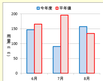
降水量の今年度と平年値の比較(アメダス大町)
