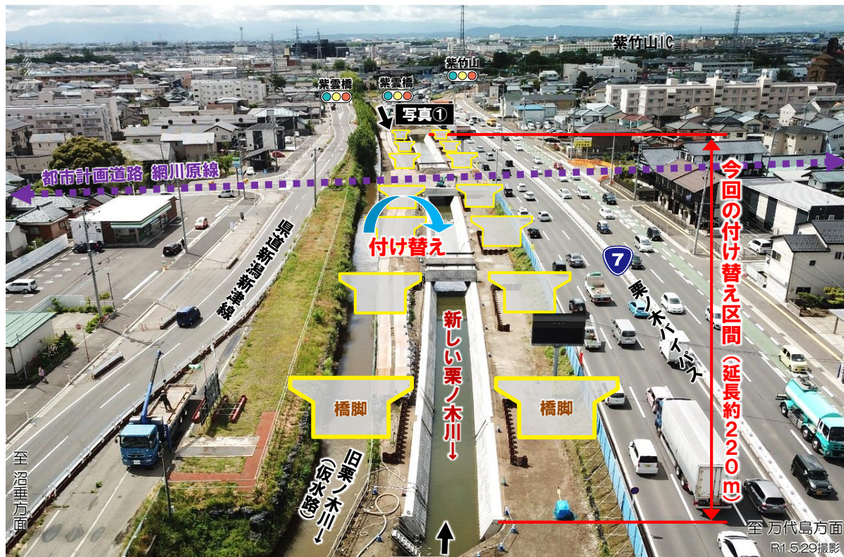
写真② ※上記の写真は川の切替え前に撮影したもので、橋脚の形はイメージです。
