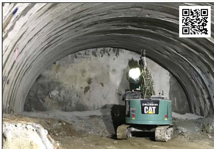
(仮称)1号トンネル貫通の瞬間 (新潟側より撮影)
