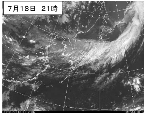
気象衛星赤外画像(東京管区気象台資料)
