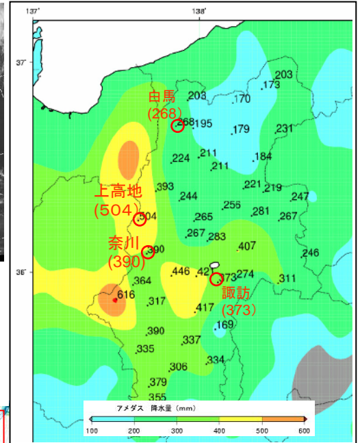
降水量分布図 H18.7.15 6h~7.19 15h (東京管区気象台資料)
