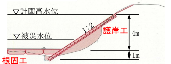
【断面図】(A-A')
