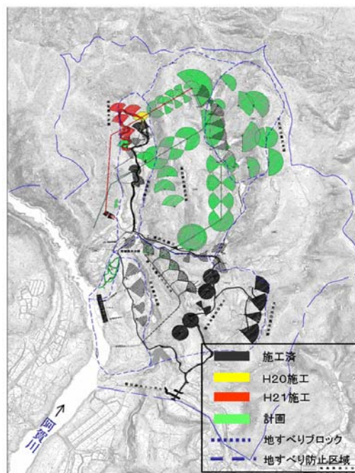
滝坂地すべり全体計画
