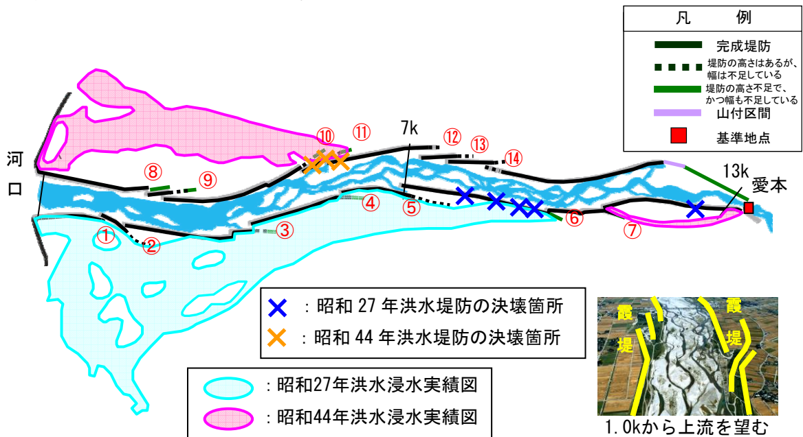
図 3-15 昭和 27 年洪水及び昭和 44 年洪水の浸水実績図と震堤の位置
