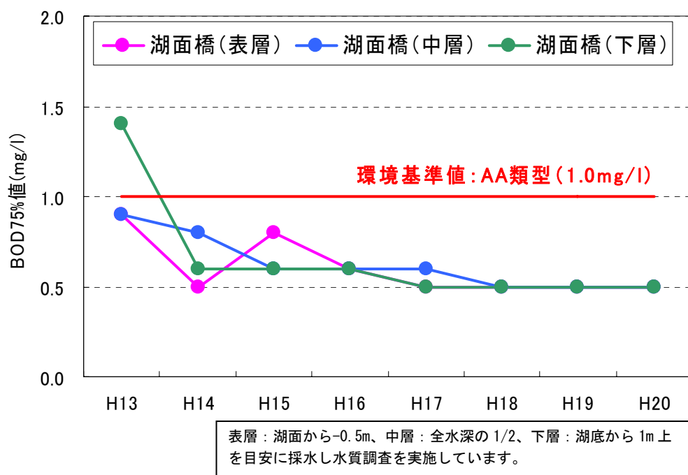
図 3-25 宇奈月ダム（湖面橋）における BOD75%値の経年変化
