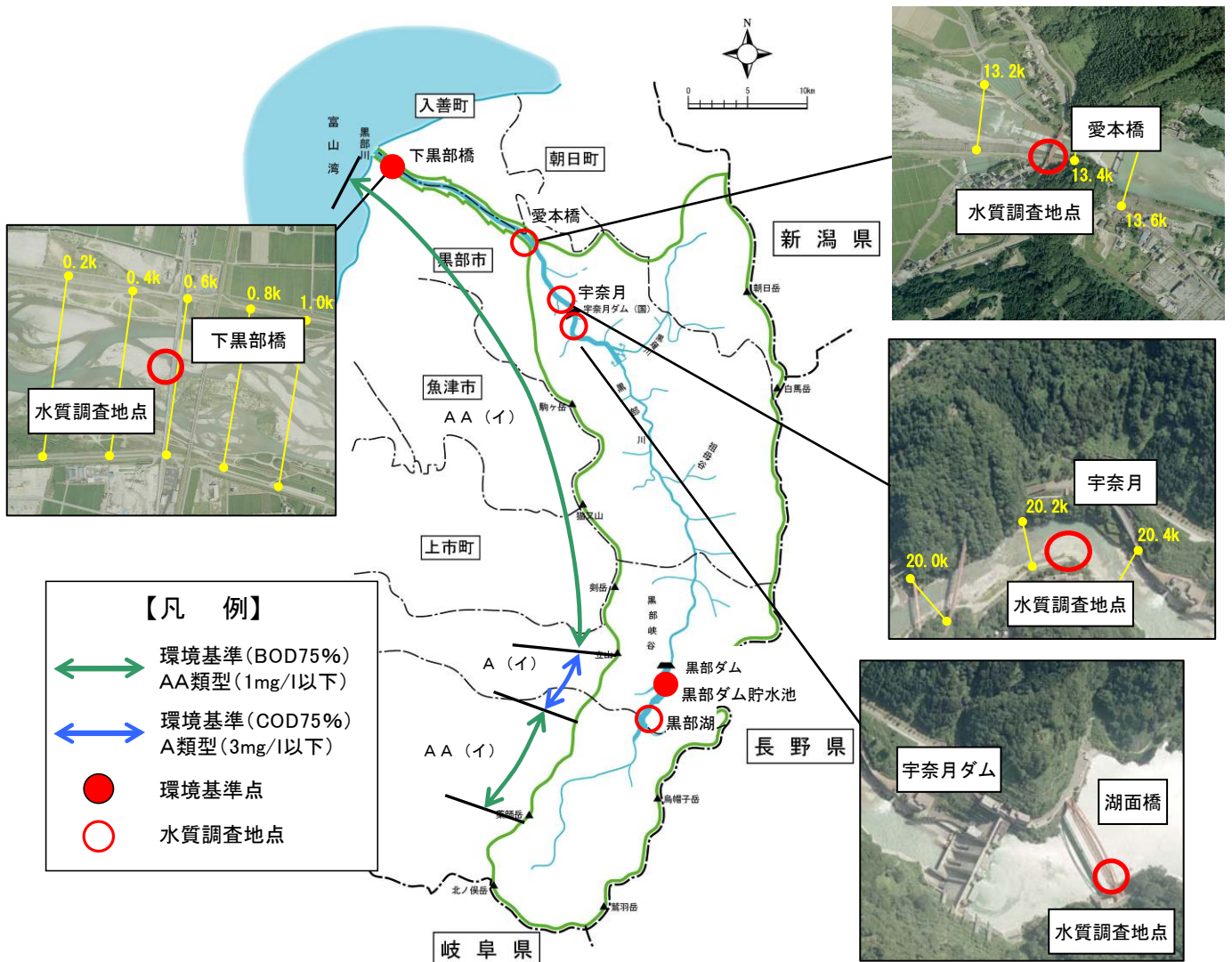
図 3-22 黒部川流域における環境基準類型指定区分及び水質調査地点
