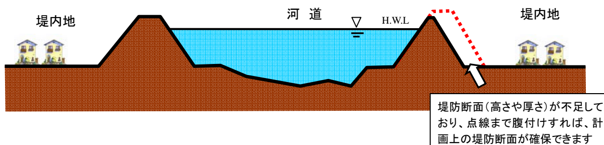
図 3-2 洪水を流下させるための堤防断面（高さや厚さ）の不足
