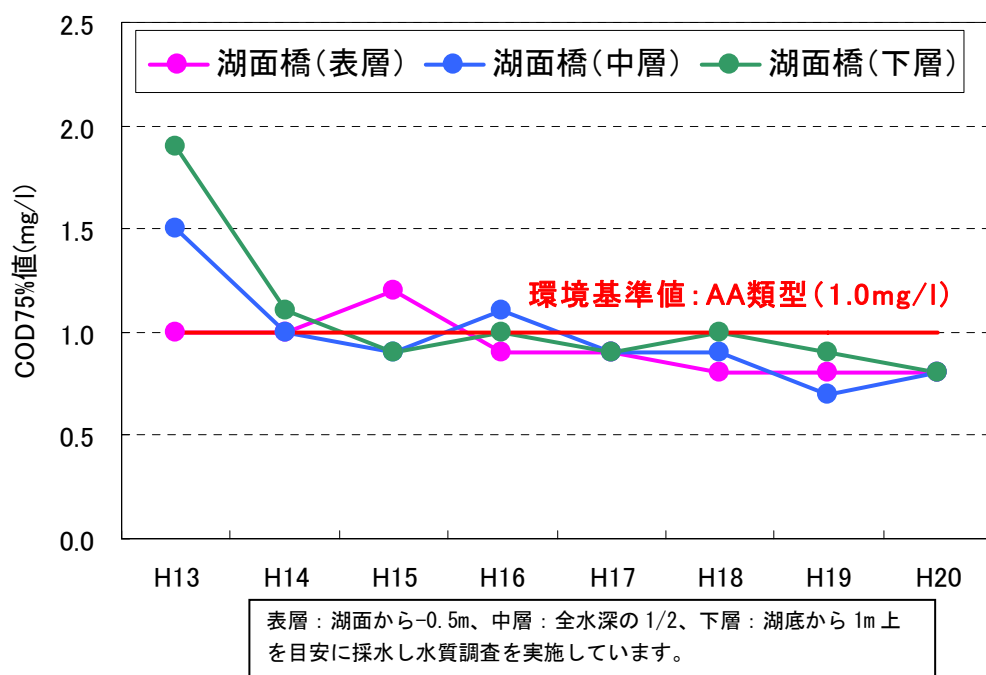
図 3-26 宇奈月ダム（湖面橋）における COD75%値の経年変化
