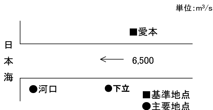
図 2-1 計画高水流量配分図
