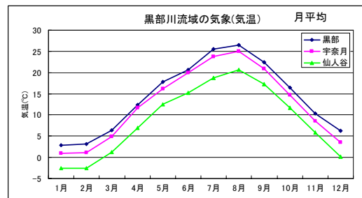
図 2-9 月平均気温
