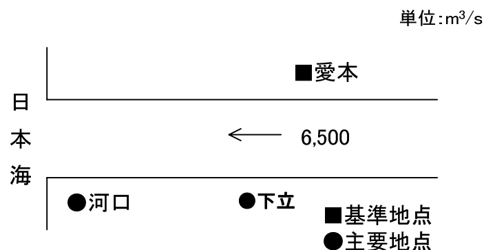
図 2-1 計画高水流量配分図
