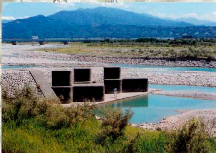
⑤ピストル水制
