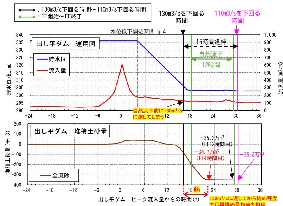
図-6 排砂シミュレーション結果
