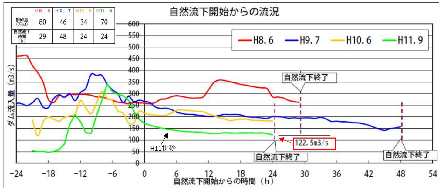
図-2 出し平ダム自然流下開始からの流況(H11排砂時) (第8回黒部川ダム排砂評価委員会(H13.3.30開催)資料抜粋)
