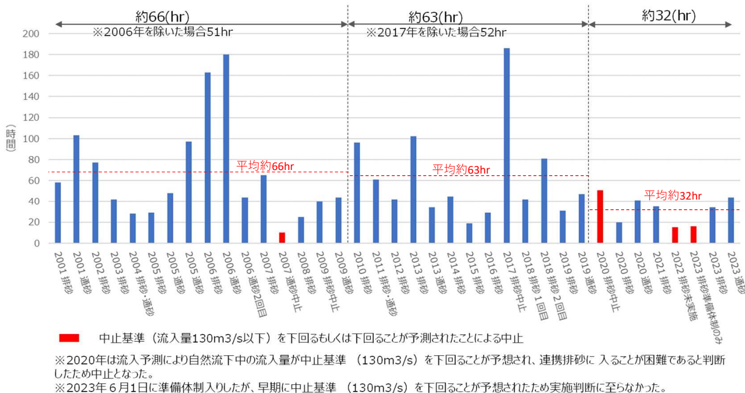
図-1 ピーク流量から中止基準流量(130m 3 /s)を下まわるまでの時間(出し平ダム)
