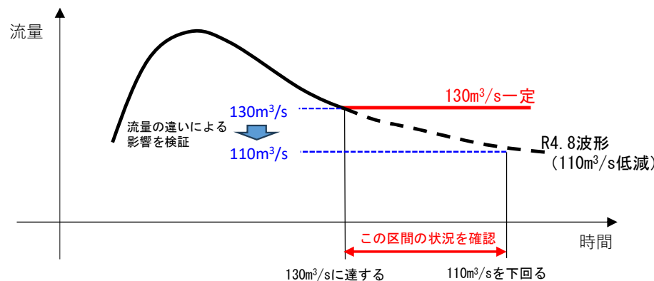
図-7 シミュレーションによる検証イメージ(項目2)
