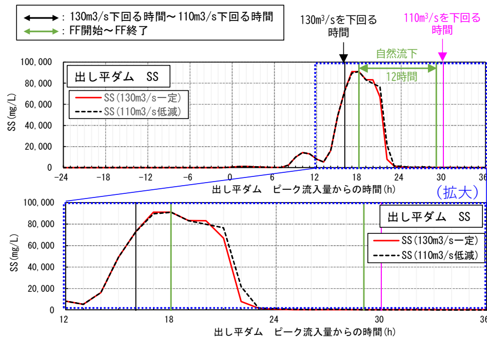
図-8 排砂シミュレーション結果(出し平ダム)
