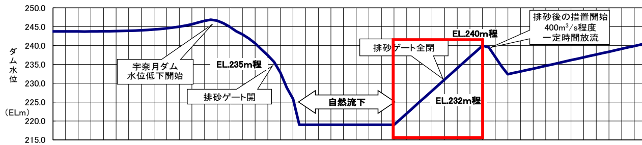
図-11 宇奈月ダム運用模式図 水位回復時間を検証
