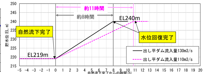
図-12 水位回復状時間
