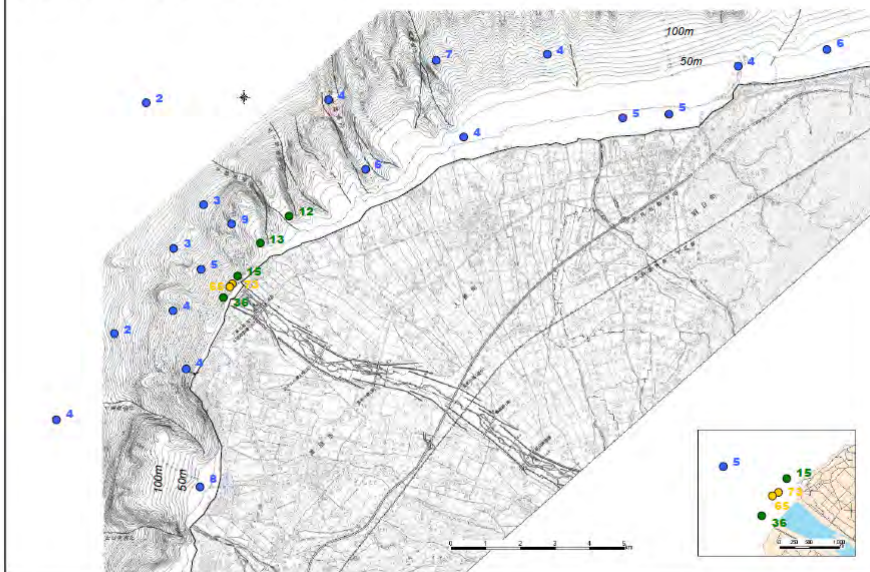
SS (7月13日12時頃)【宇奈月ダム：通砂後の措置開始前】
