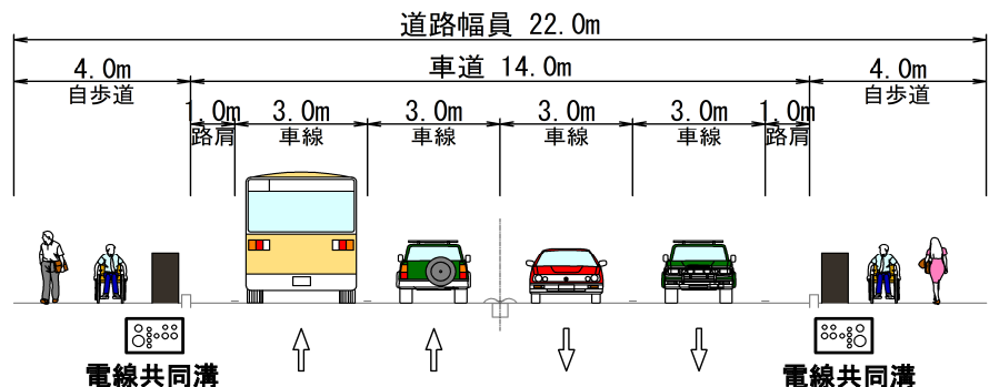
<計画断面図>
