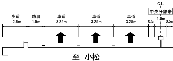
整備後 (3車線)
