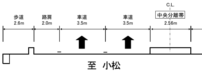
整備前 (2車線)
