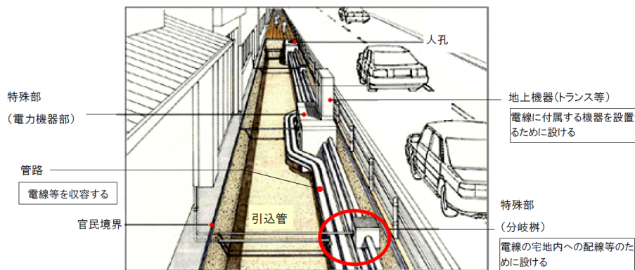
【電線共同溝の基本構造】
