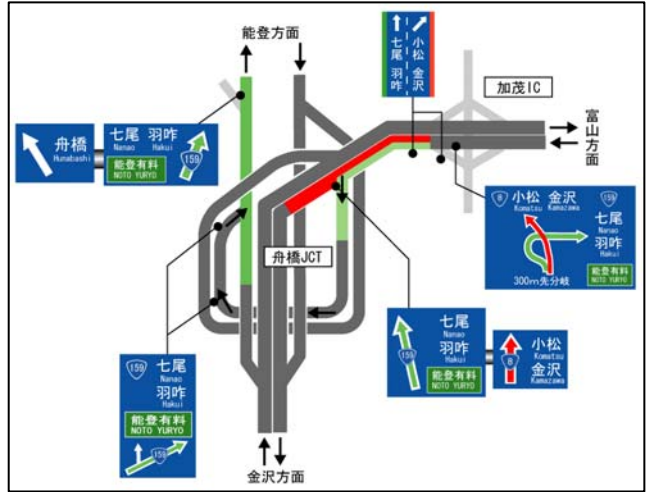
舟橋ジャンクション概要図
