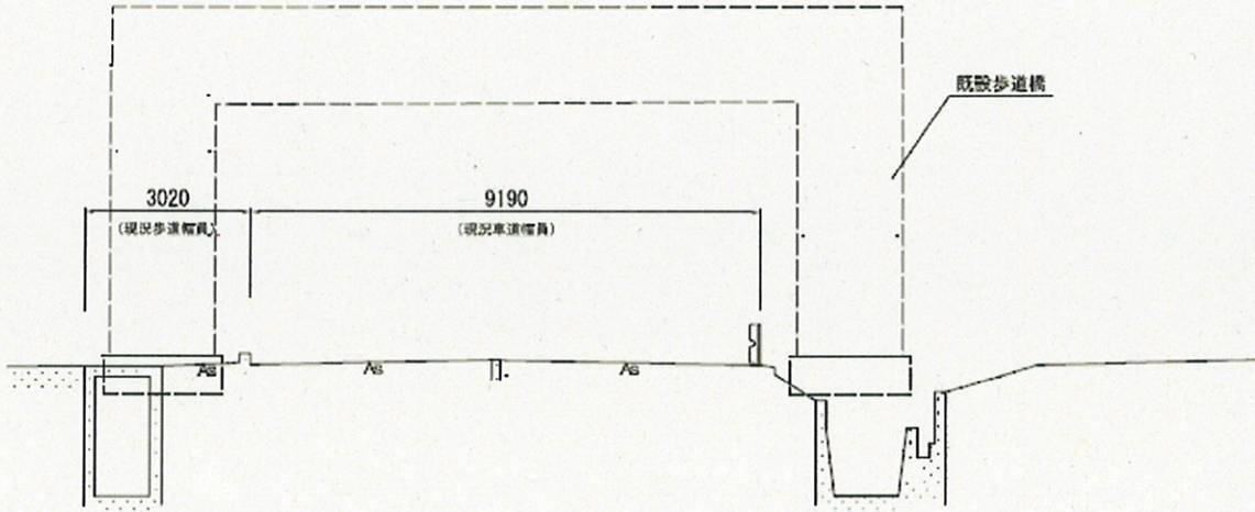
現況断面図
