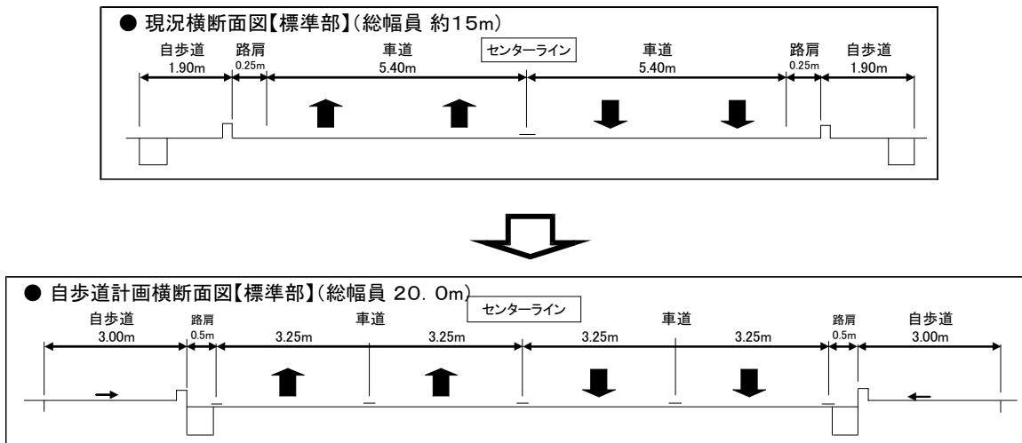
【横断面図】
