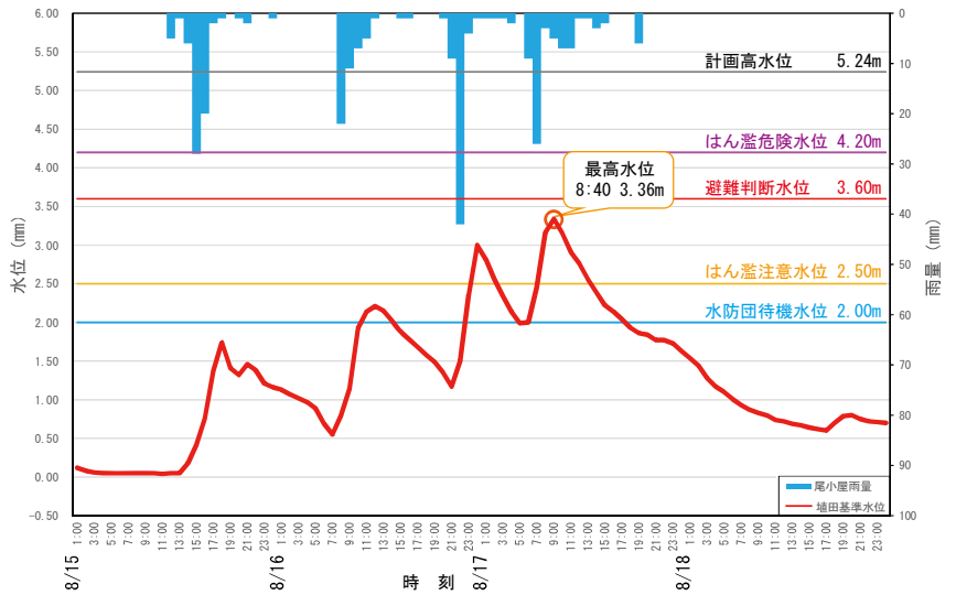
平成 26 年 8 月 15 ~ 18 日 梯川流域出水ハイドログラフ
