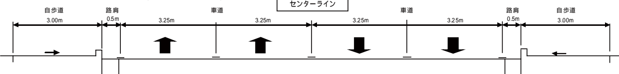
自歩道計画横断面図【標準部】(総幅員 20.0m)
