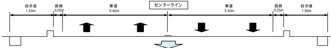
現況横断面図【標準部】(総幅員 約15m)
