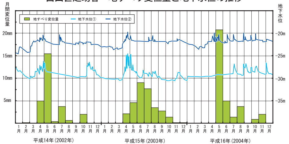
白山甚之助谷・地すべり変位量と地下水位の推移
