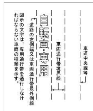
▼道路標示「専用通行帯（109の6）」
