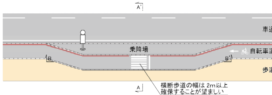
【A-A' 断面】
