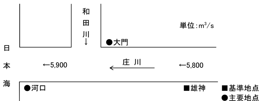
図 2.2.4 庄川水系河川整備基本方針計画高水流量配分図
