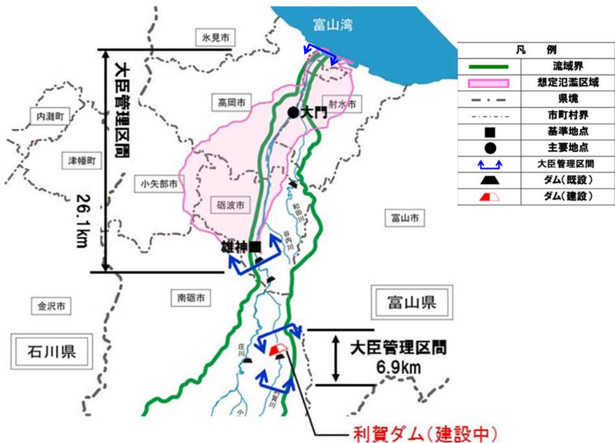
図 2.1.7 雄神・大門地点位置図
