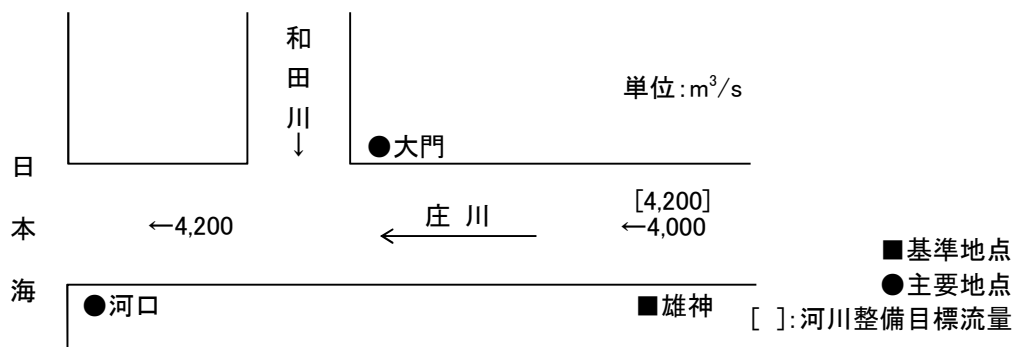
図 2.2.5 庄川水系河川整備計画河道配分図
