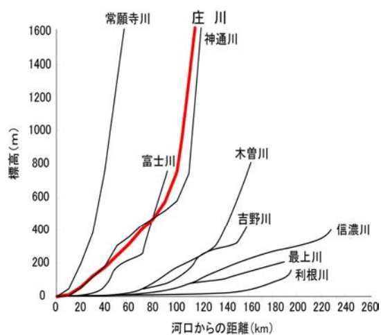
図 2.1.3 河床勾配の比較
