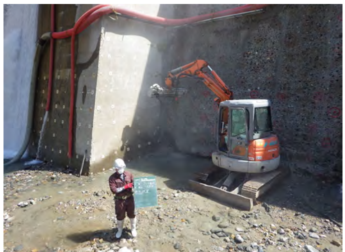
削孔状況
