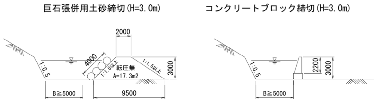
断面図
