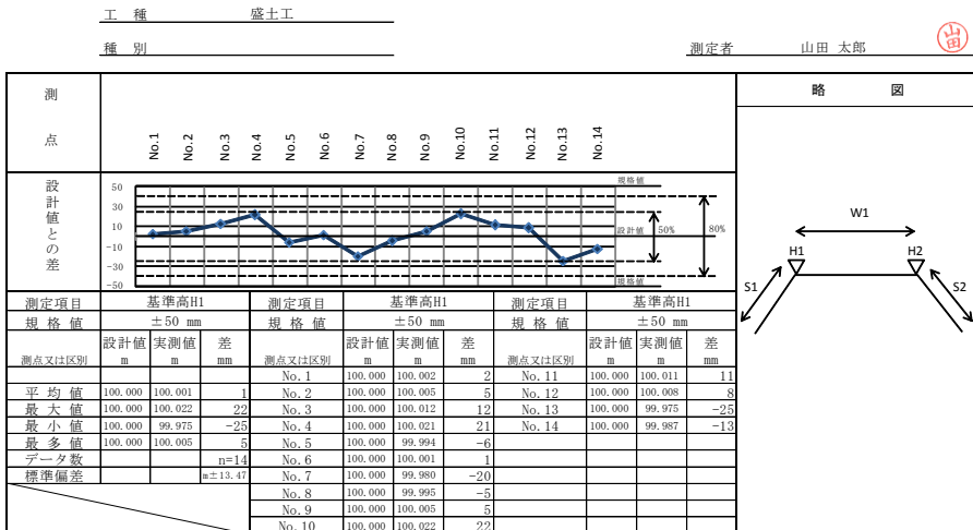
図-3 作成帳票例 (出来形管理図表)
