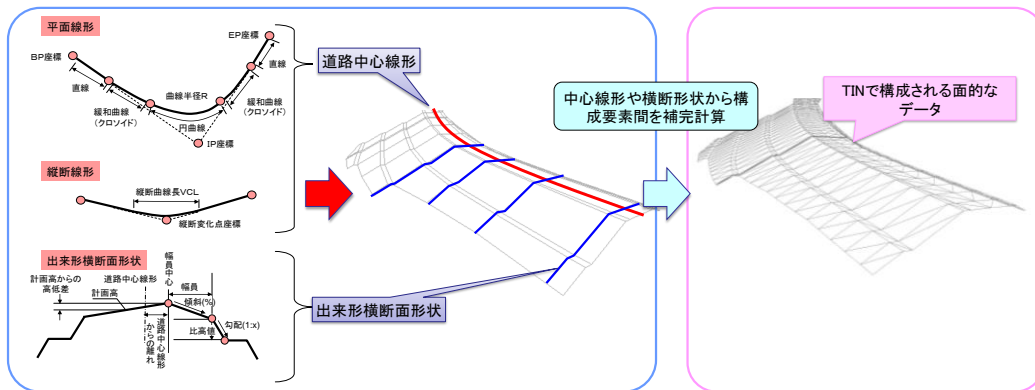
図 3次元設計データと作成するために必要な構成要素
