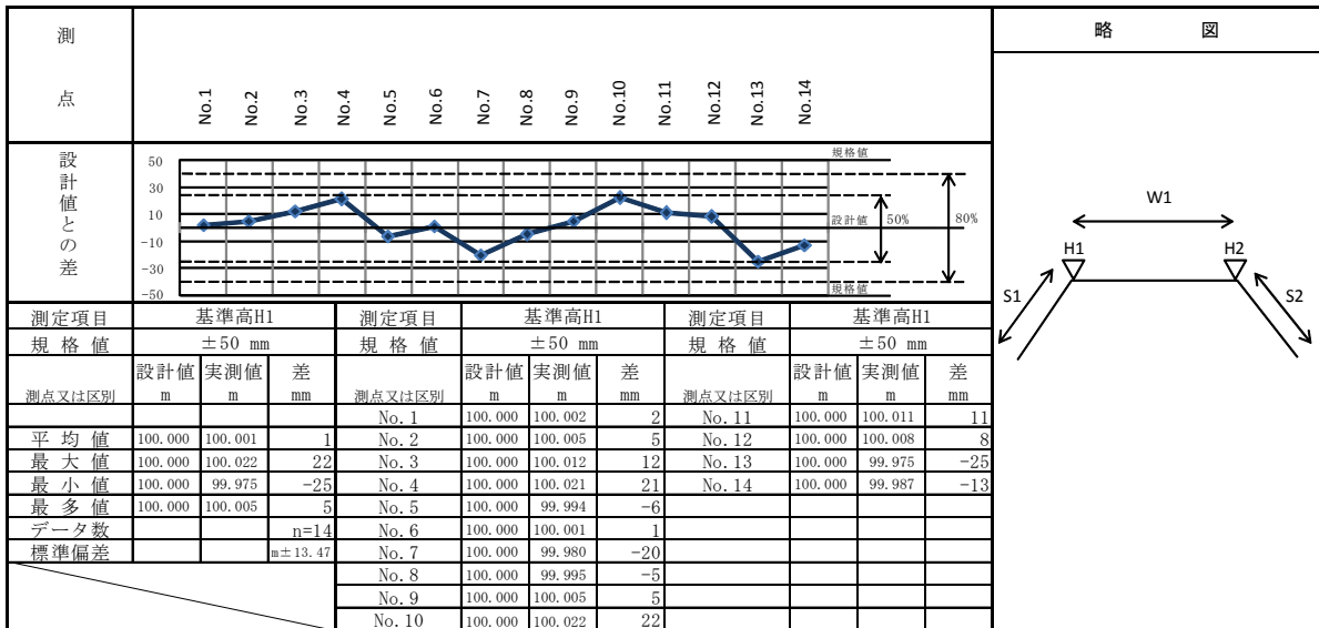
図-3 作成帳票例 (出来形管理図表)
