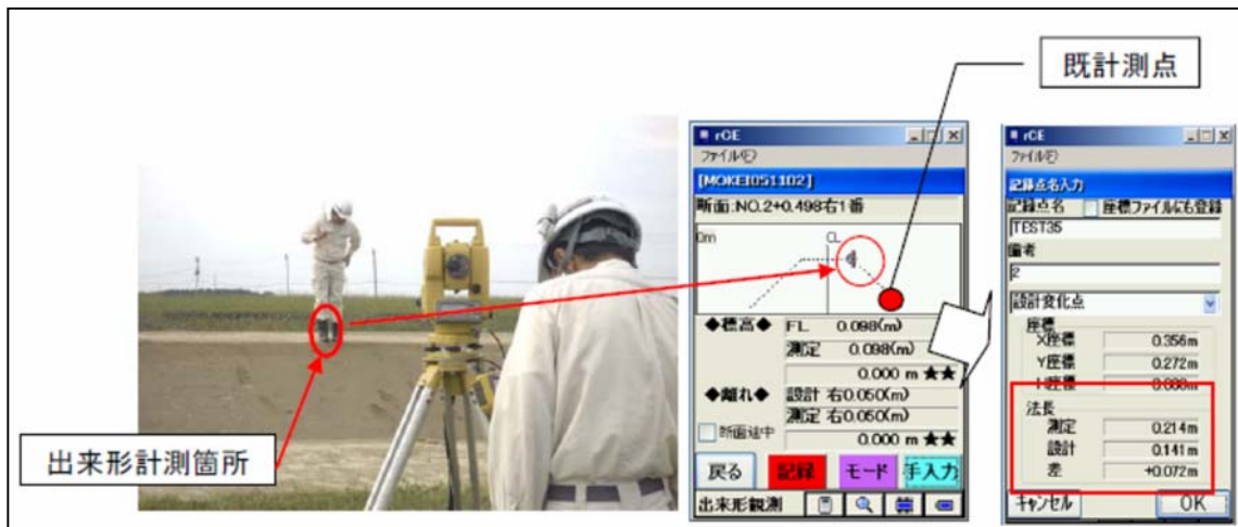
図-5 出来形計測状況及び現場確認画面例
