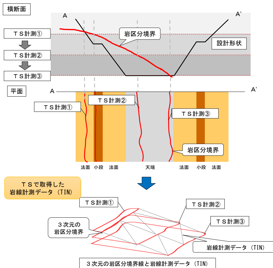
図 1-18 TSで取得する岩区分境界のイメージ
