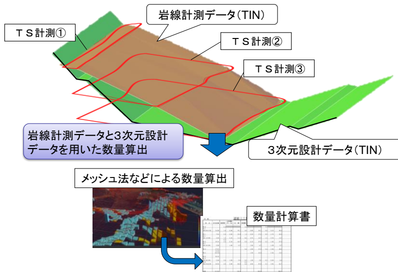
図 1-17 設計変更（岩区分）のための数量算出イメージ
