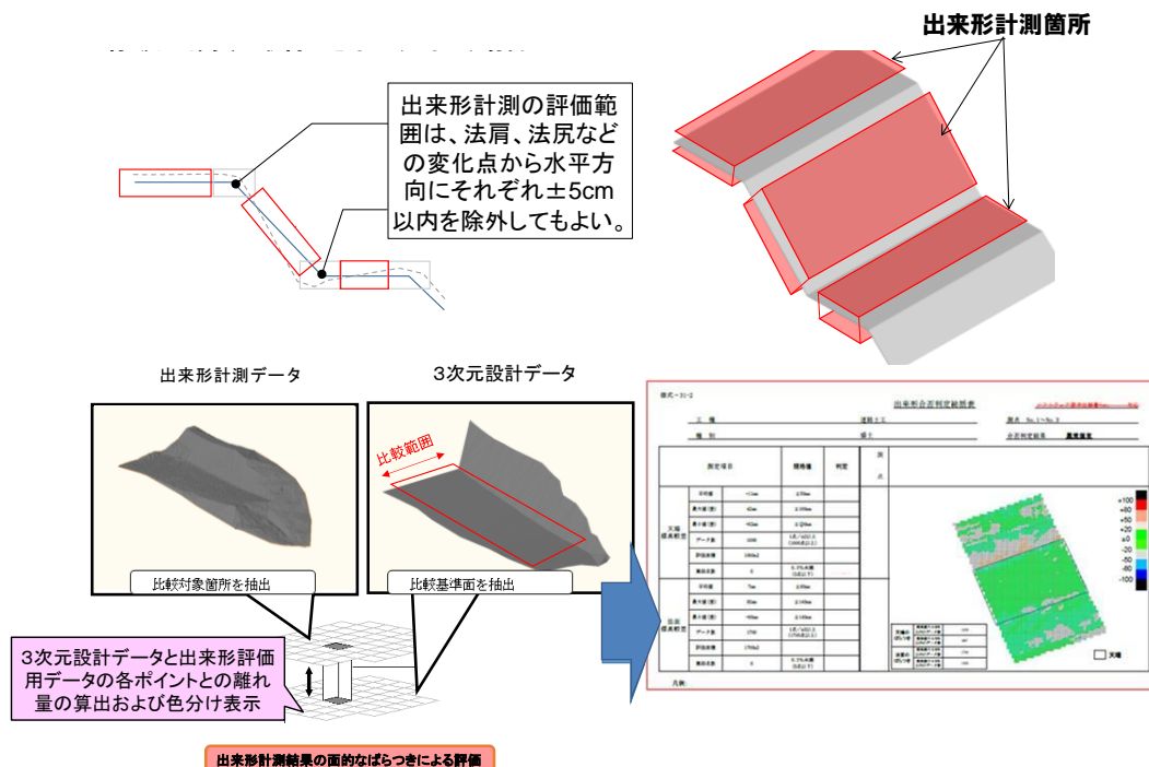
図 1-23 出来形管理図表 作成の流れ
