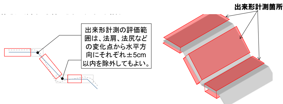
図 2-6 出来形計測箇所
