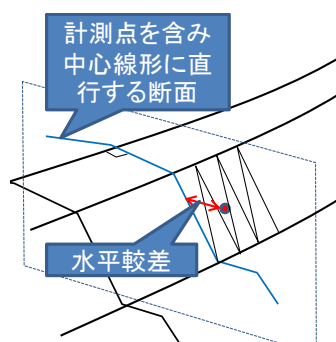
図 1-13 水平較差の算出ロジックのイメージ
