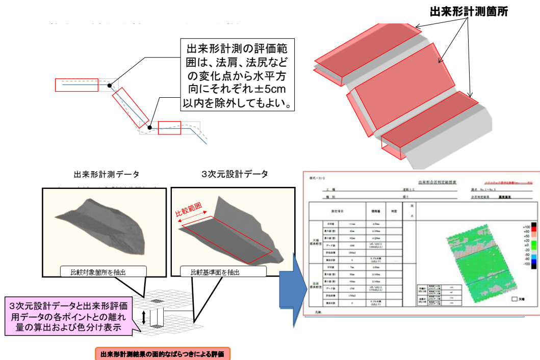
図 1-15 面的な出来形管理分布図のイメージ
