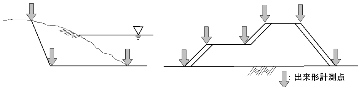
図 2-5 出来形計測箇所
