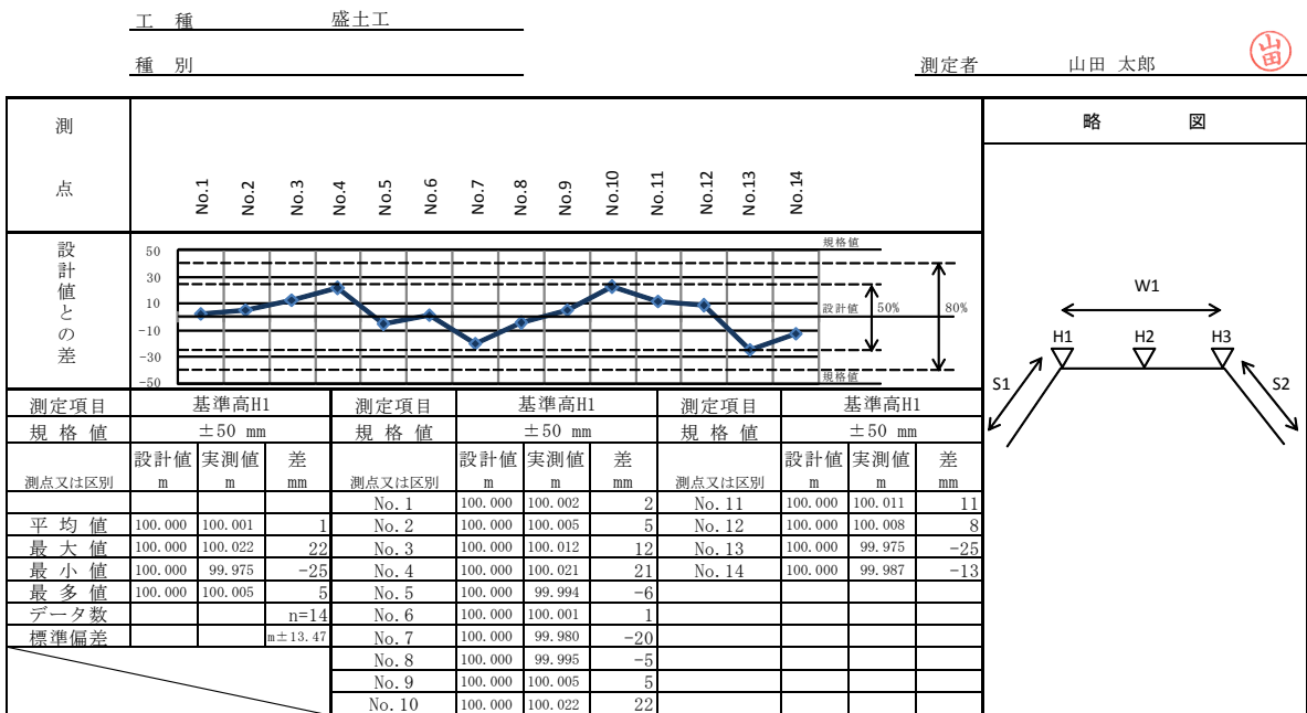
図 1-22 出来形管理図表 作成例
