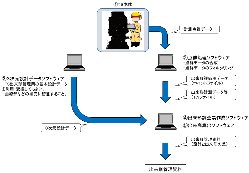
図 1-10 出来形管理用 TS による出来形管理機器の構成例 (面管理の場合)
