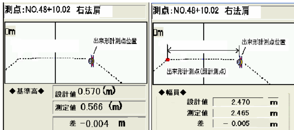
図 1-11 出来形管理用TSによる出来形確認画面例
