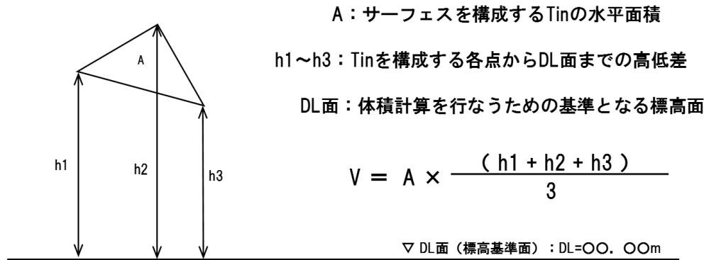
図 1-28 TIN分割等を用いた求積による数量算出
