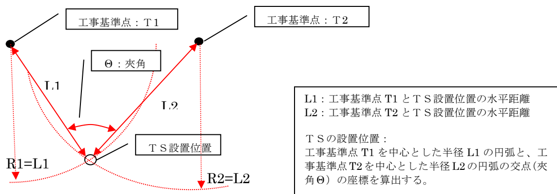
図 1-8 後方交会法での器械位置算出 (例)
