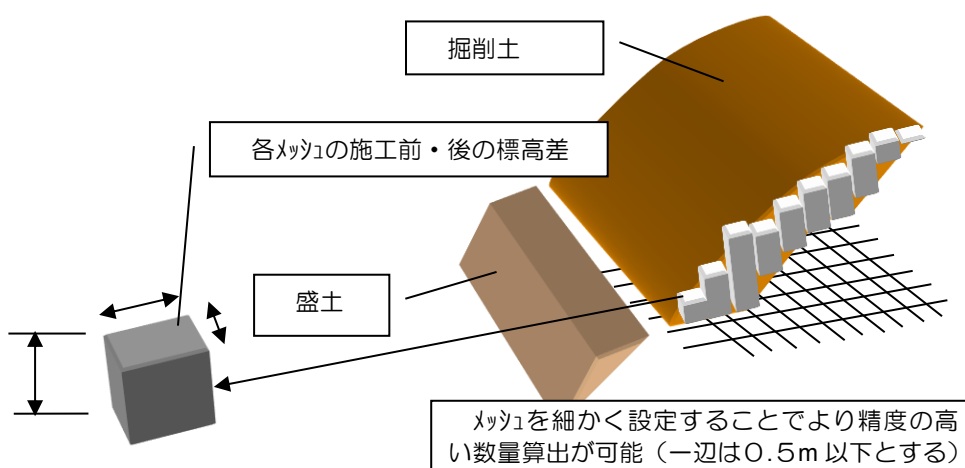
図 1-26 メッシュ法による数量算出の条件と適用イメージ
