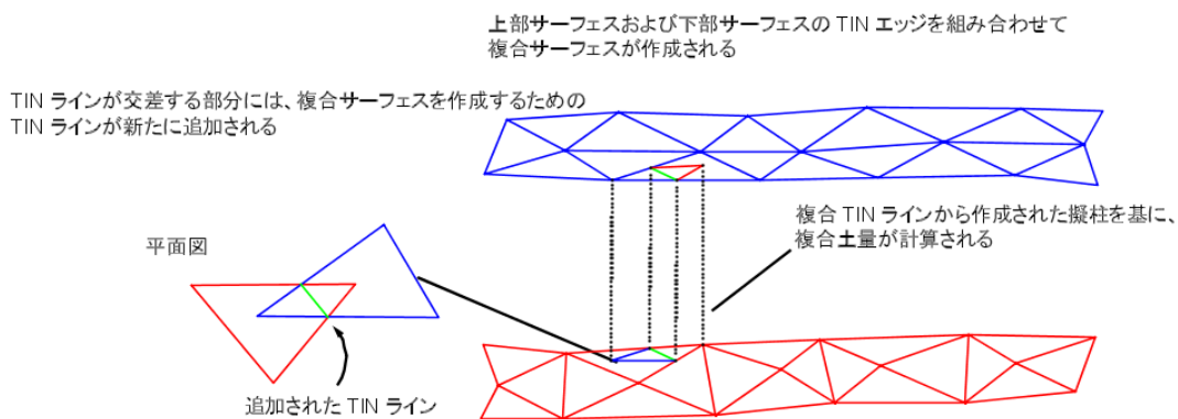
図 1-29 プリズモイダル法による数量算出
