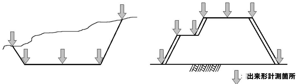
図 2-1 出来形計測箇所
