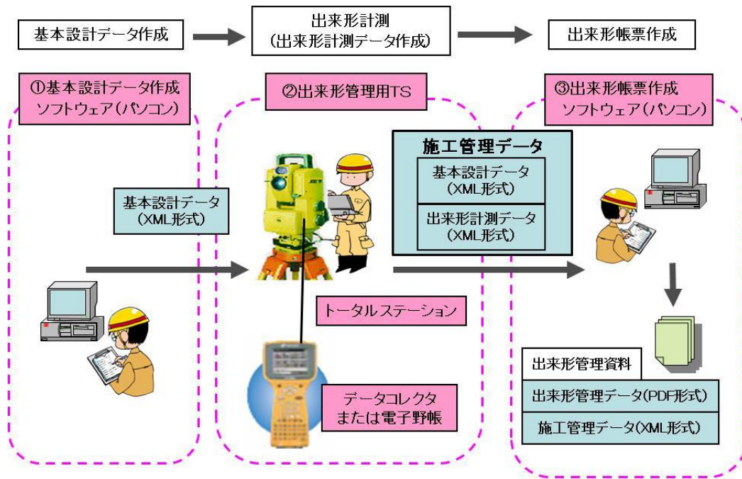
図 1-9 出来形管理用 TS による出来形管理機器の構成例
