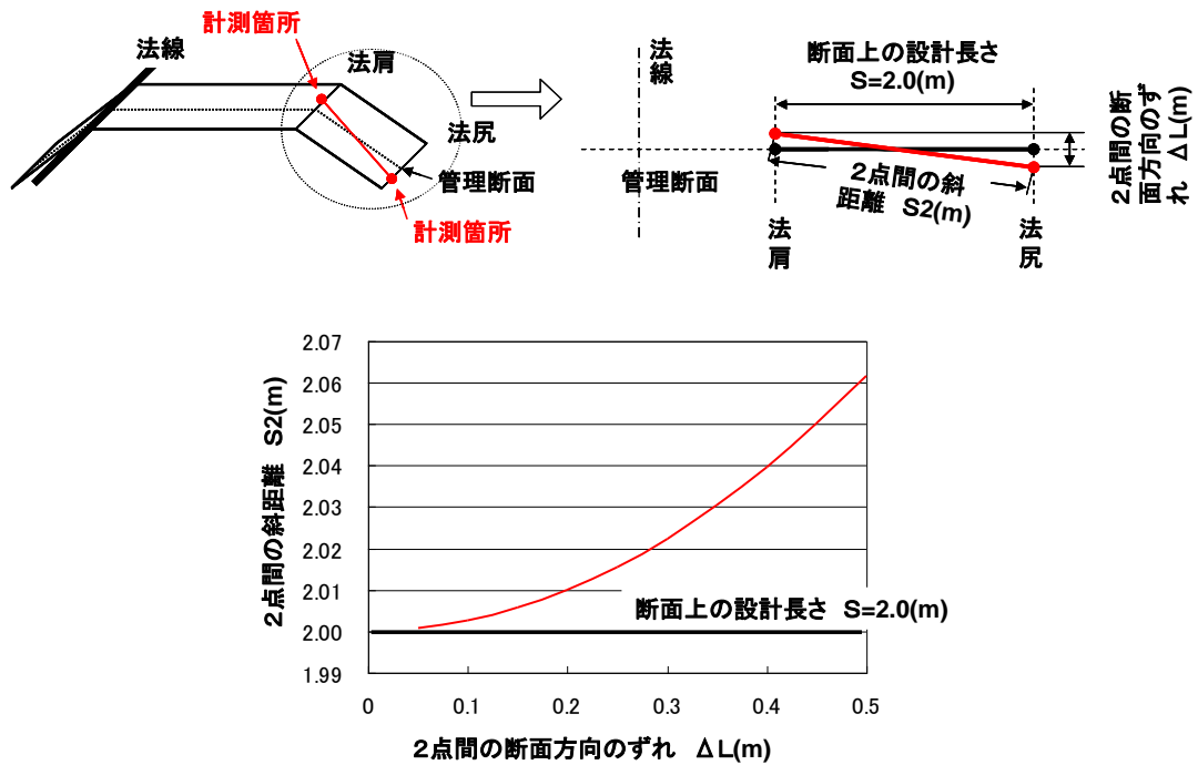
図 2-7 管理断面上の出来形計測点誤差が及ぼす長さ誤差の影響範囲
