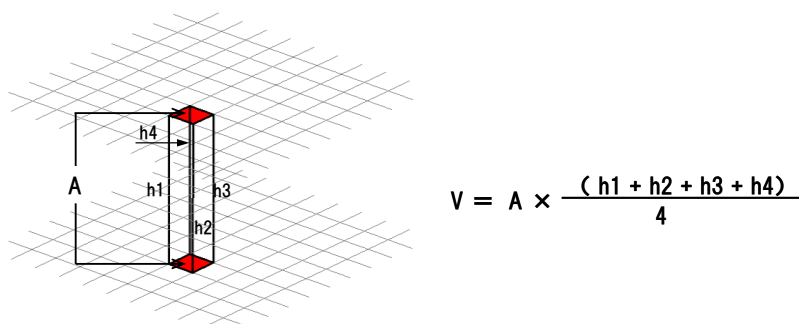
図 1-27 点高法による数量算出
