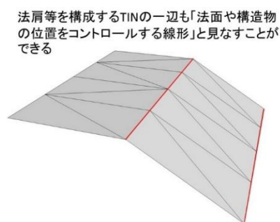
図 1-14 位置をコントロールする線形
