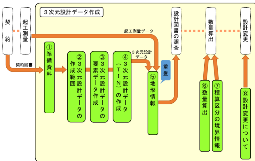
図 1-20 3次元設計データの流れ
