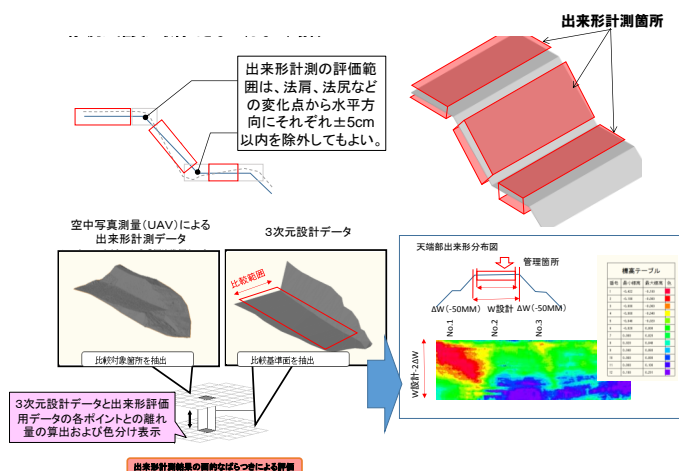
図 1-17 出来形管理図表 作成の流れ
