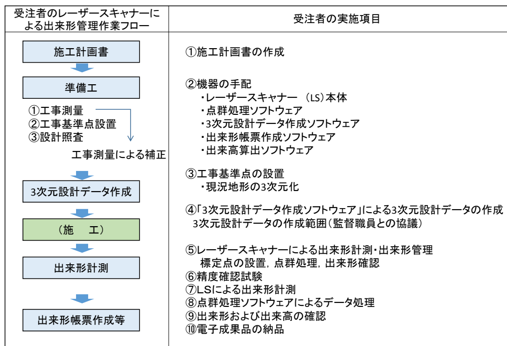
図 1-1 LSによる計測の手順
