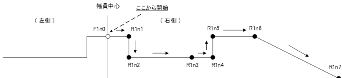
図 16 完成形状の構成点を記述する順序のイメージ
