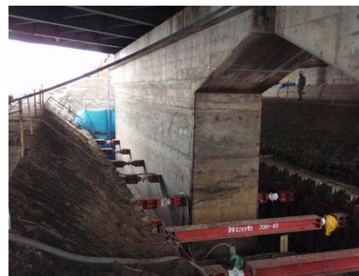
変更後の鋼矢板土留工
