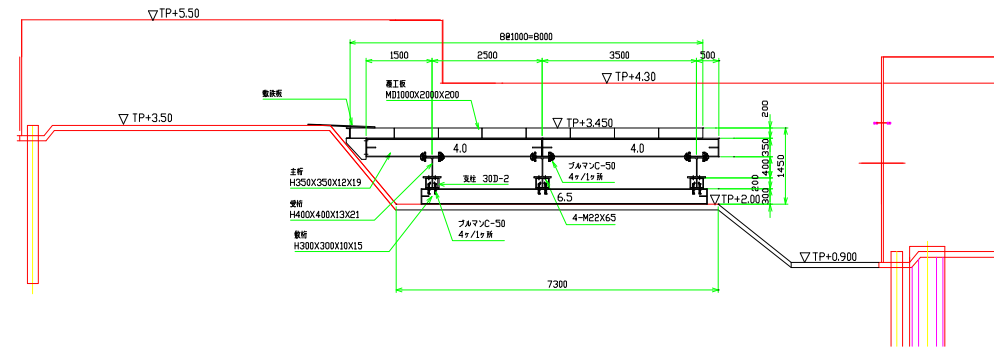
作業構台
