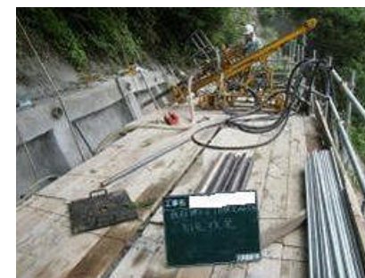
ケーシング併用による削孔
