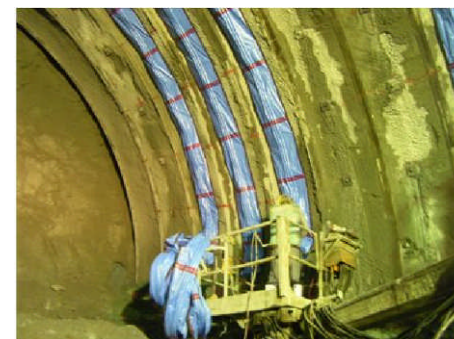
湧水処理施工状況
