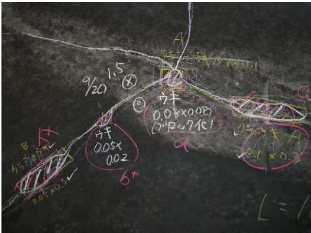
トンネル内壁のひび割れ状況
