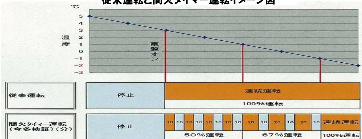
従来運転と間欠タイマー運転イメージ図
