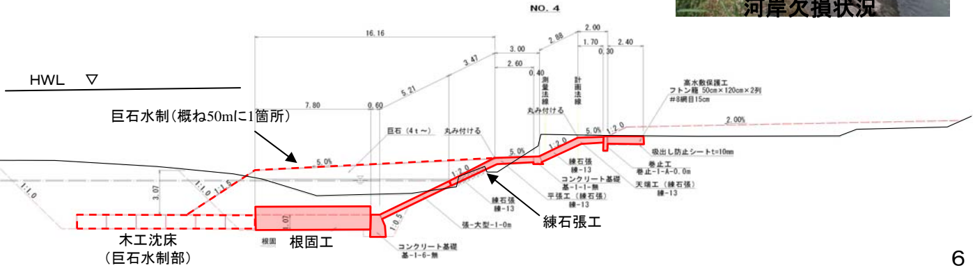
護岸工断面図
